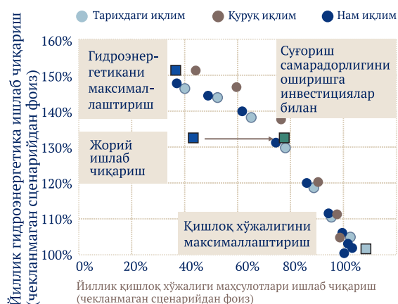
5.6-расм. Сув омборлари каскадининг мувофиқлаштирилган ва оптималлаштирилган иши ҳозирда ҳам, иқлим ўзгариши шароитида ҳам сув ва энергетика хавфсизлигини таъминлашга хизмат қилади. Манба: Жаҳон банки, 2020.
